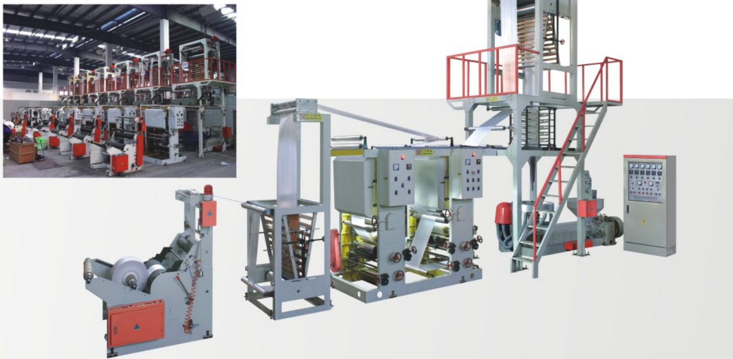
Main Technical Variables / 主要技術參數
